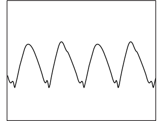
20 Vp-p (409 kHz)
